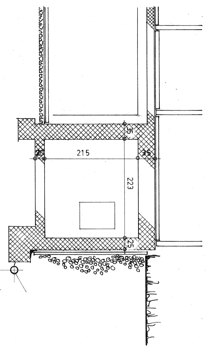
SCHNITT LUFTSCHUTTRAUM
