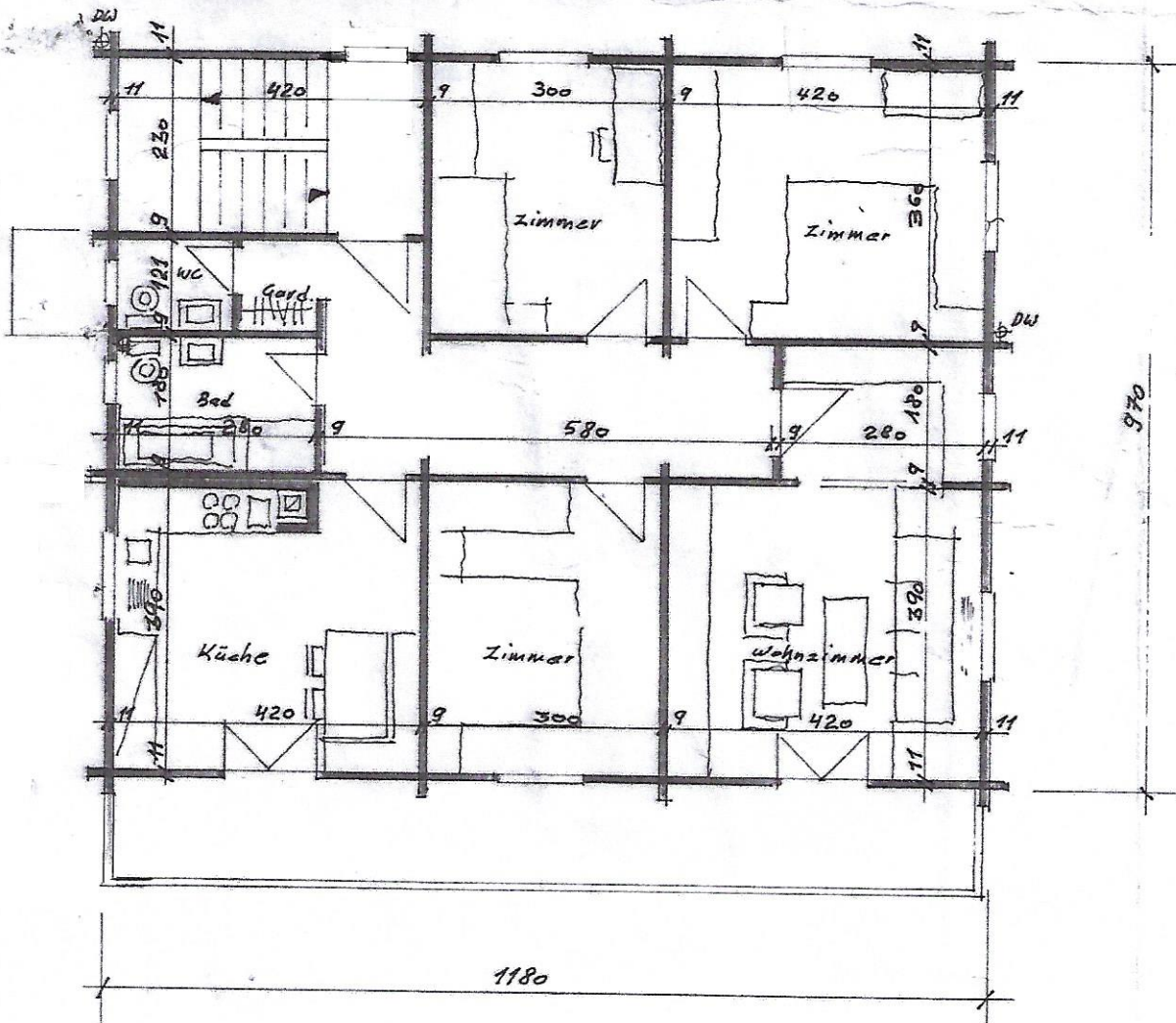
GRUNDRISS WOHNGESCHOSS 1+2
