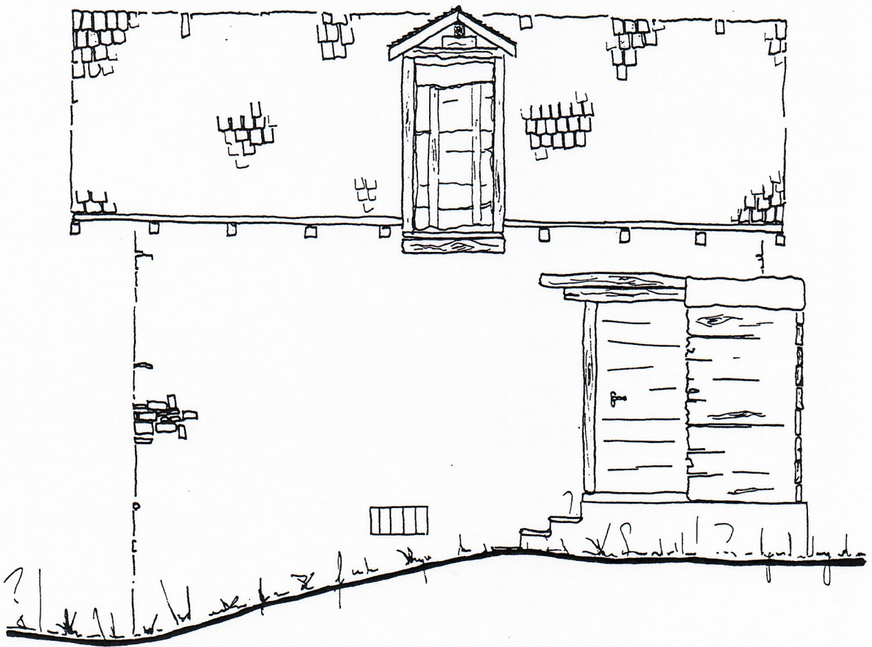
ANSICHT NORDEN
