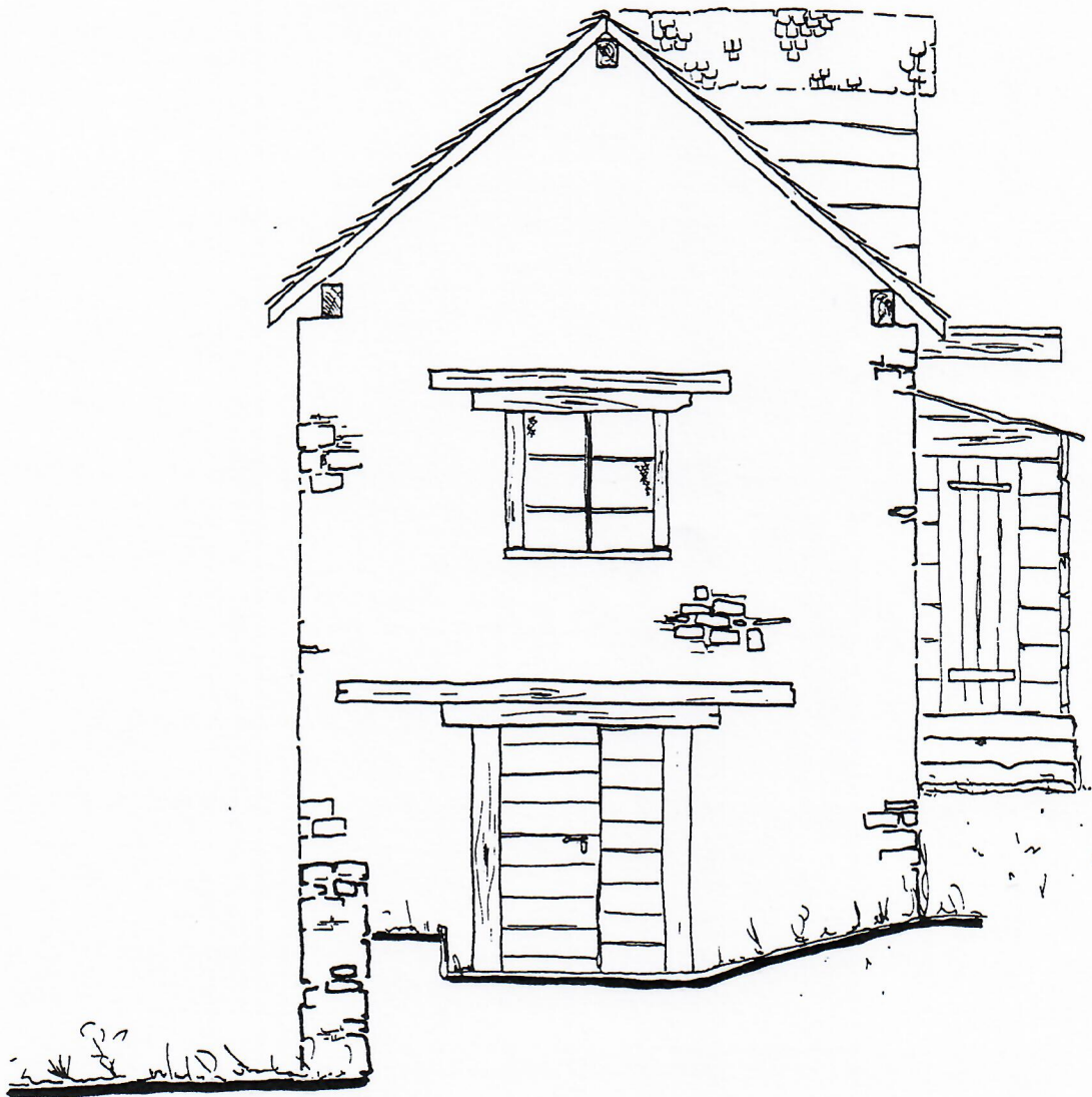
ANSICHT OSTEN
