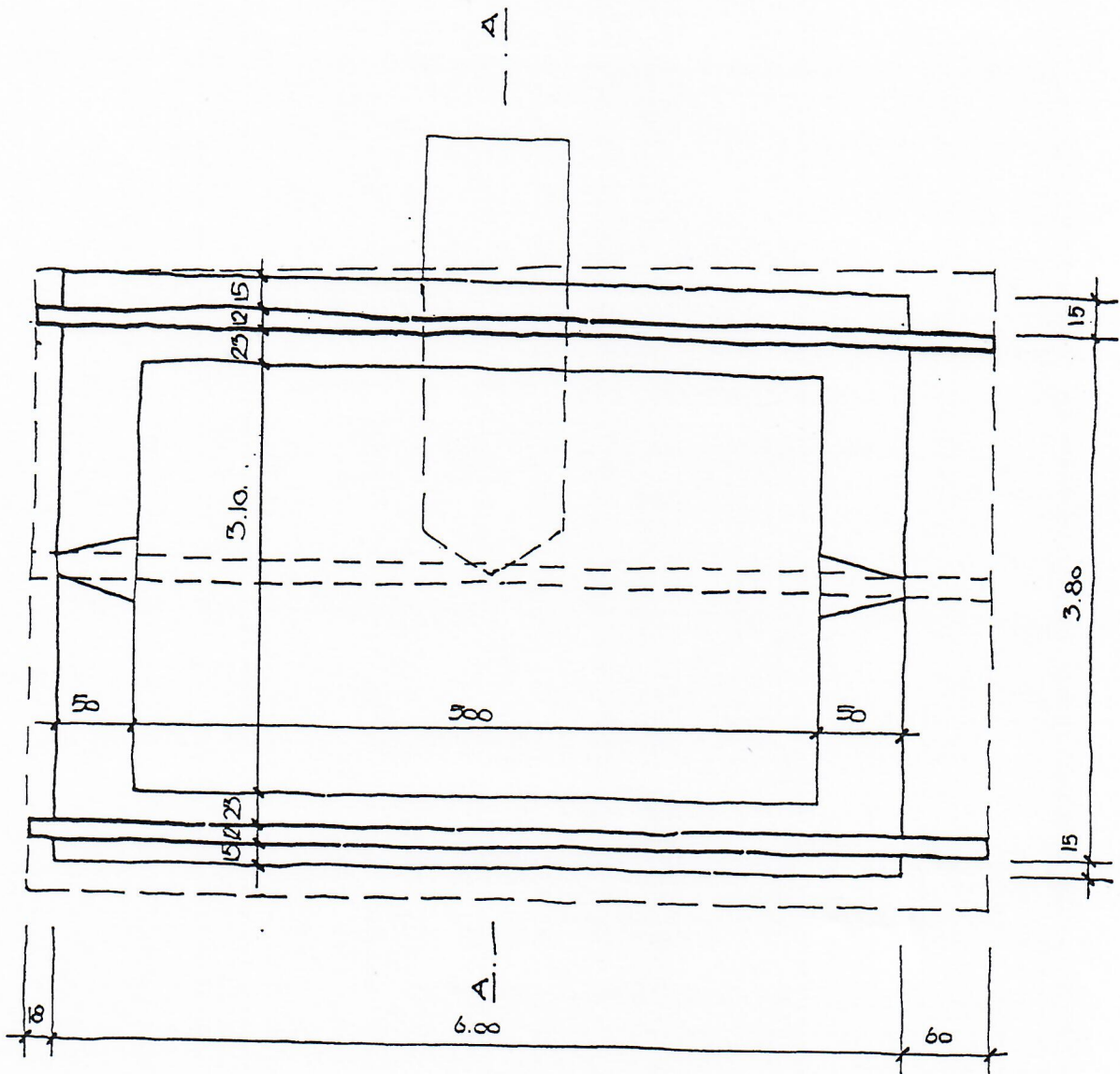
GRUNDRISS 06
