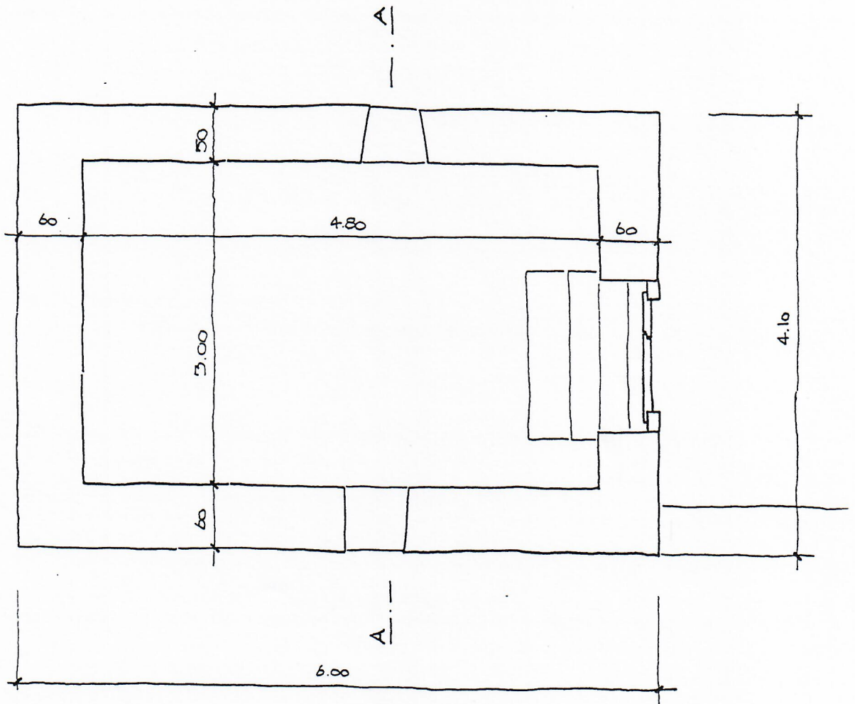
GRUNDRISS KB
