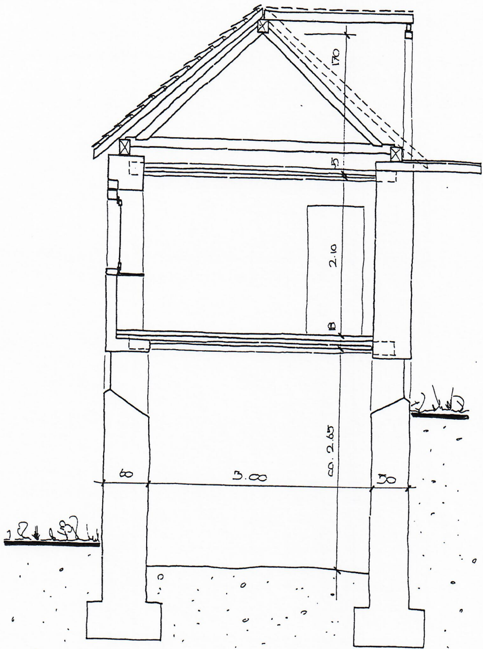
SCHNITT A--A
