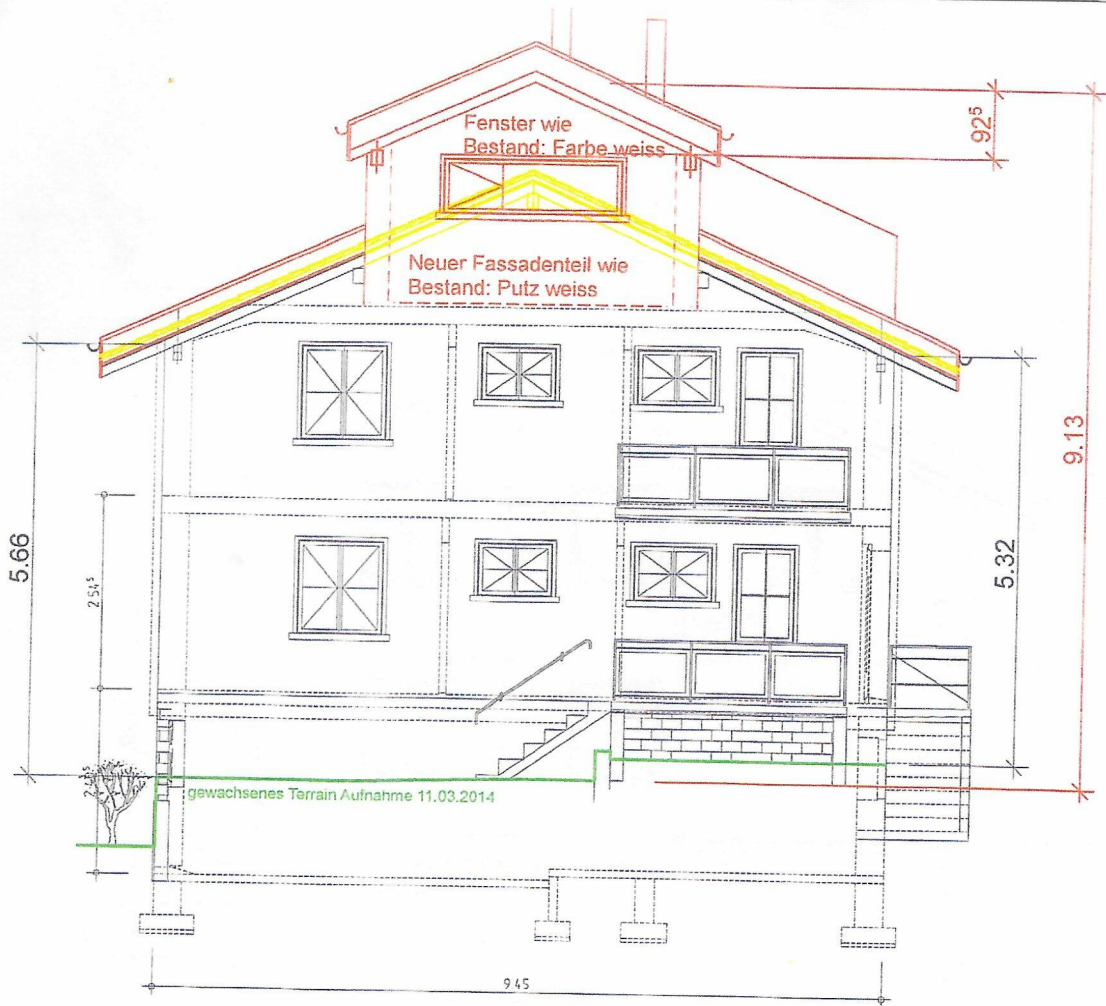
Südfassade
