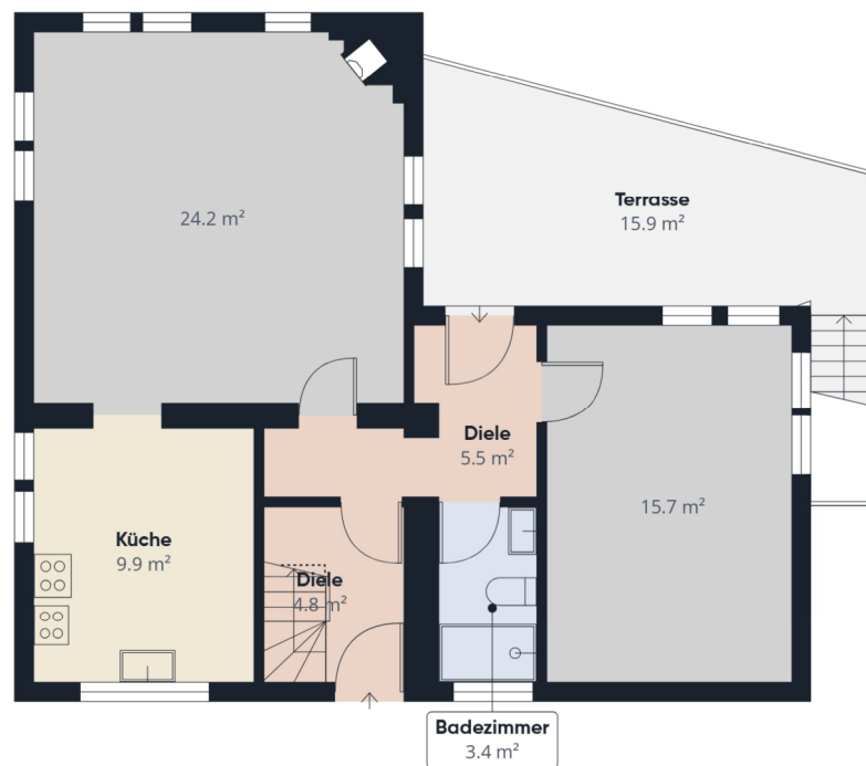
Etage 0
